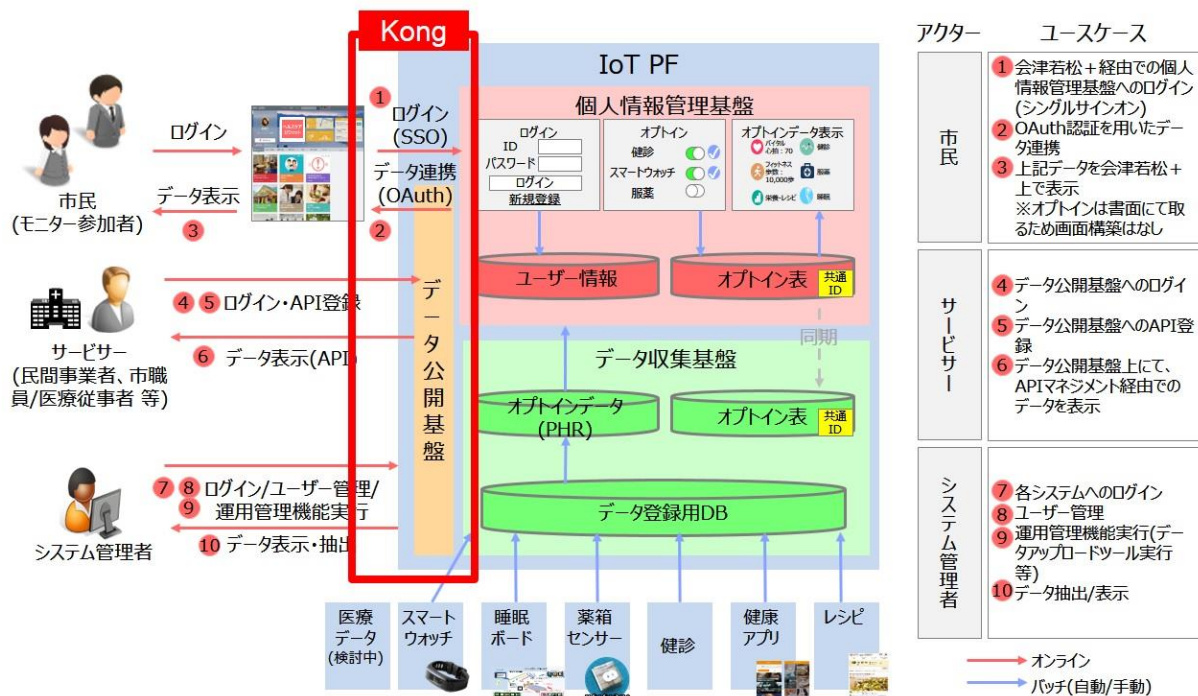
図1：会津若松市 IoT ヘルスクエアプラットフォーム事業のシステム構成図
